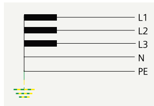
TN-S Sistem
