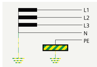
TT Sistem
